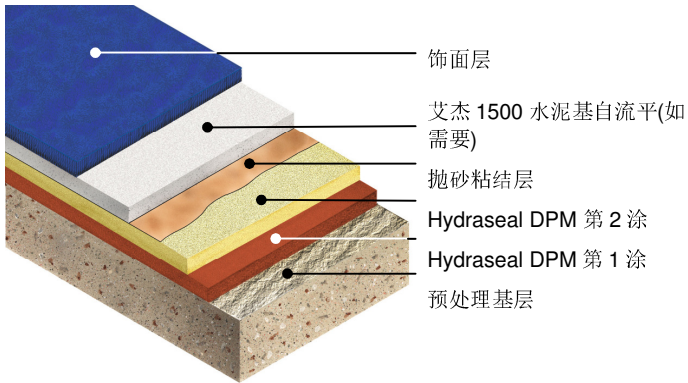
常规富杰 DPM 环氧防潮层剖面图
